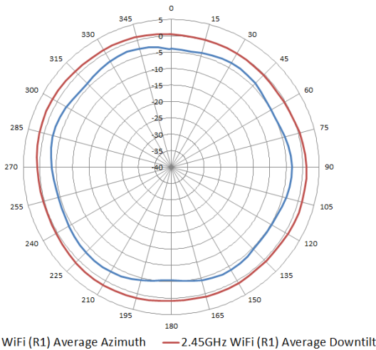
2.45 GHz Wi-Fi (antennas 0, 1, 2, 3)
