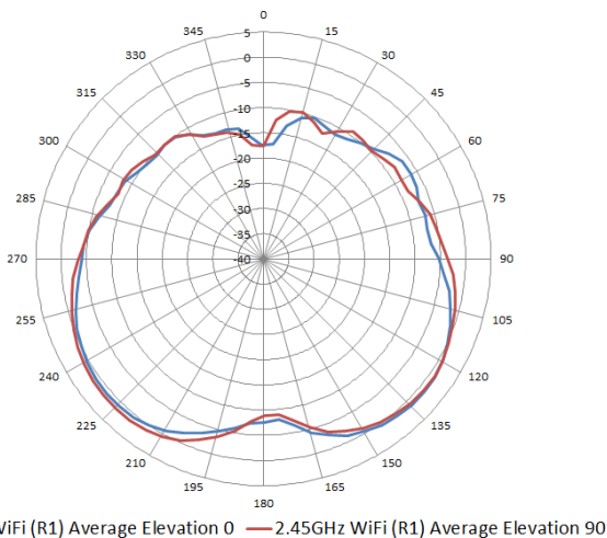
2.45 GHz Wi-Fi (antennas 0, 1, 2, 3)
