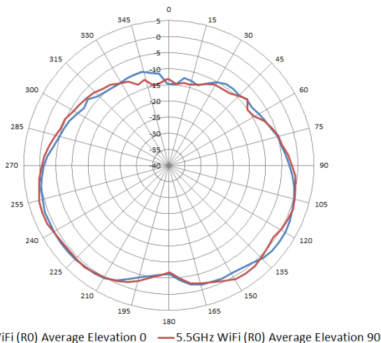
5.5 GHz Wi-Fi (antennas 0, 1, 2, 3)
