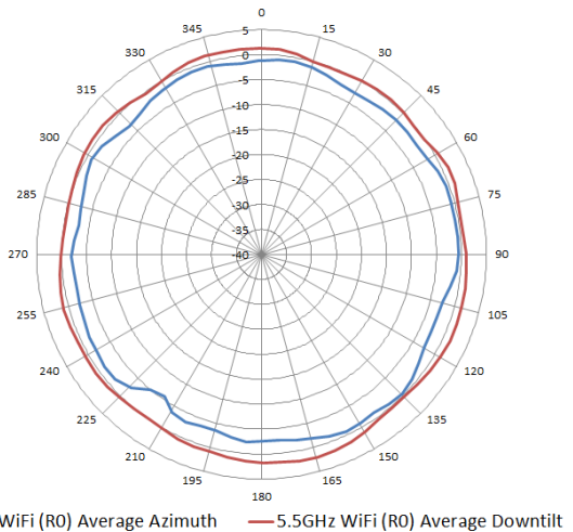
5.5 GHz Wi-Fi (antennas 0, 1, 2, 3)
